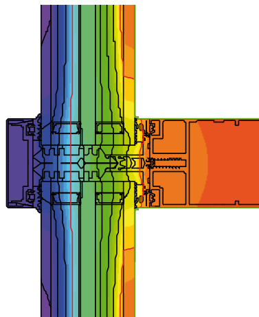
Izotermický průběh
