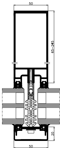
Řez sloupkem
