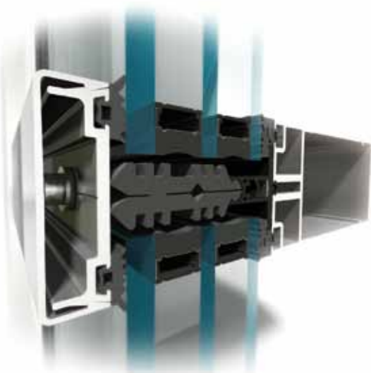
Řez příčkou
